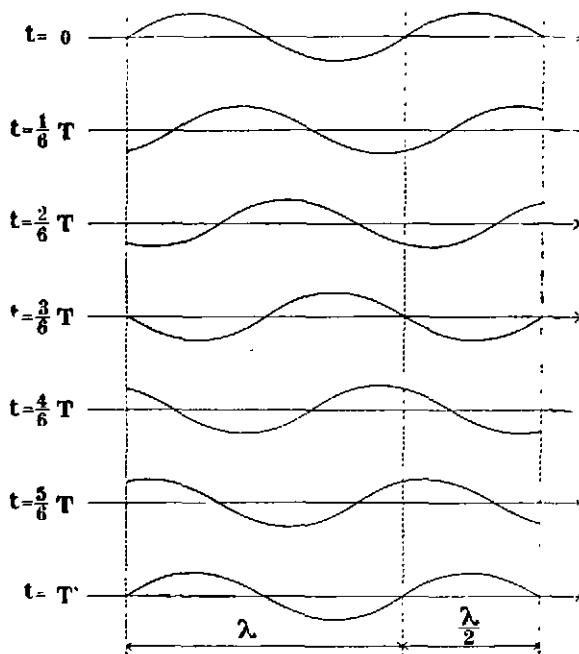
השתנות הגל במשך המחזור T ציור 2
